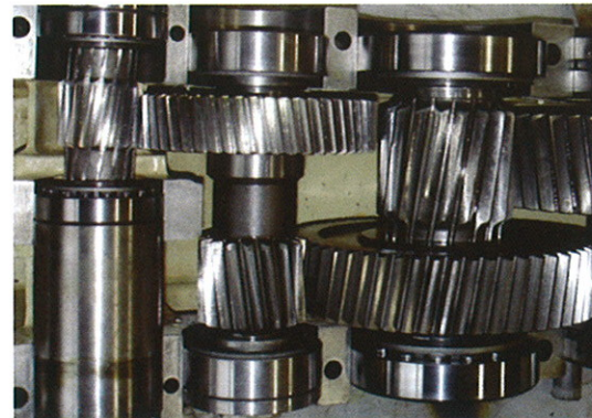
Reparatur Getriebe
